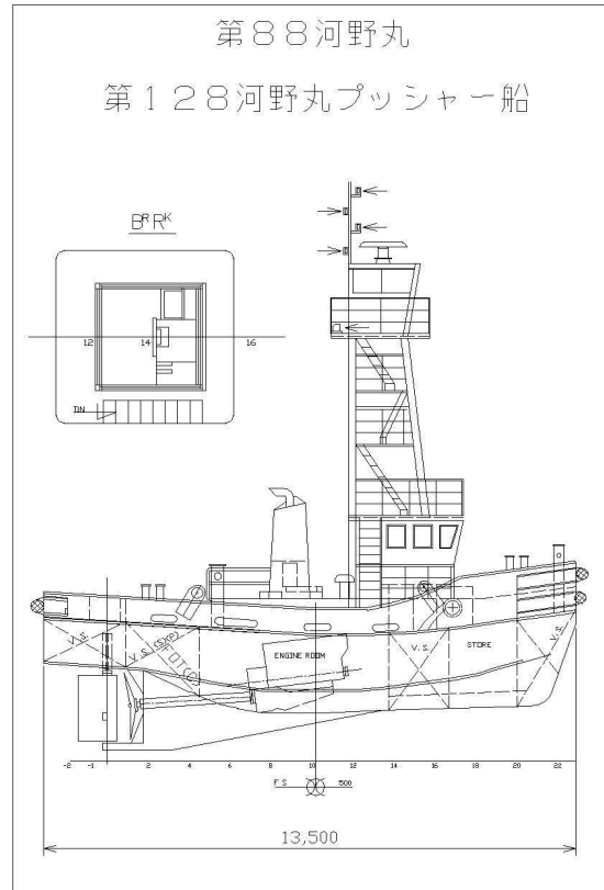
押航船 第八十八河野丸
