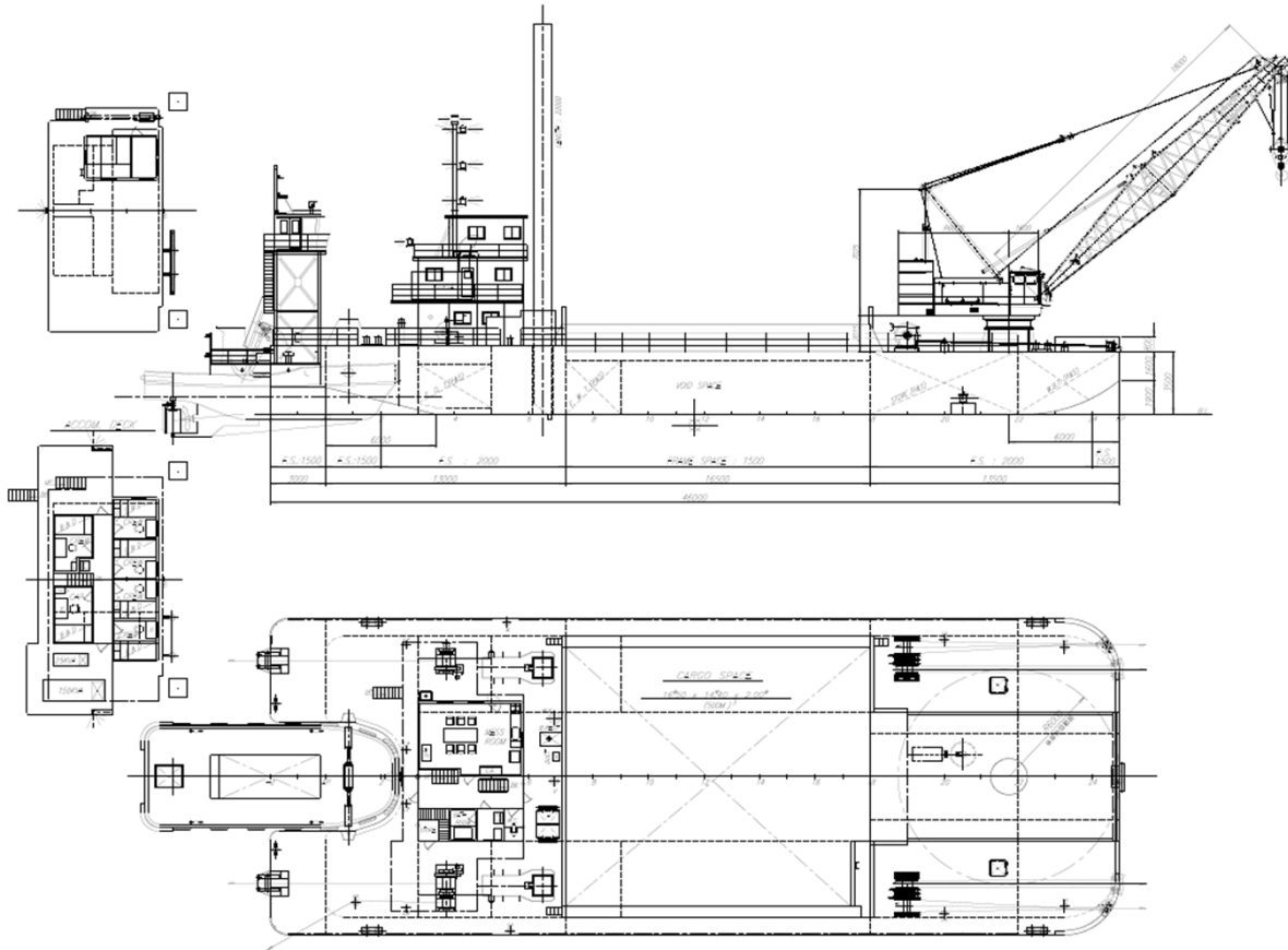
CCH2000-6F 台船搭載荷重表（縦方向吊）
